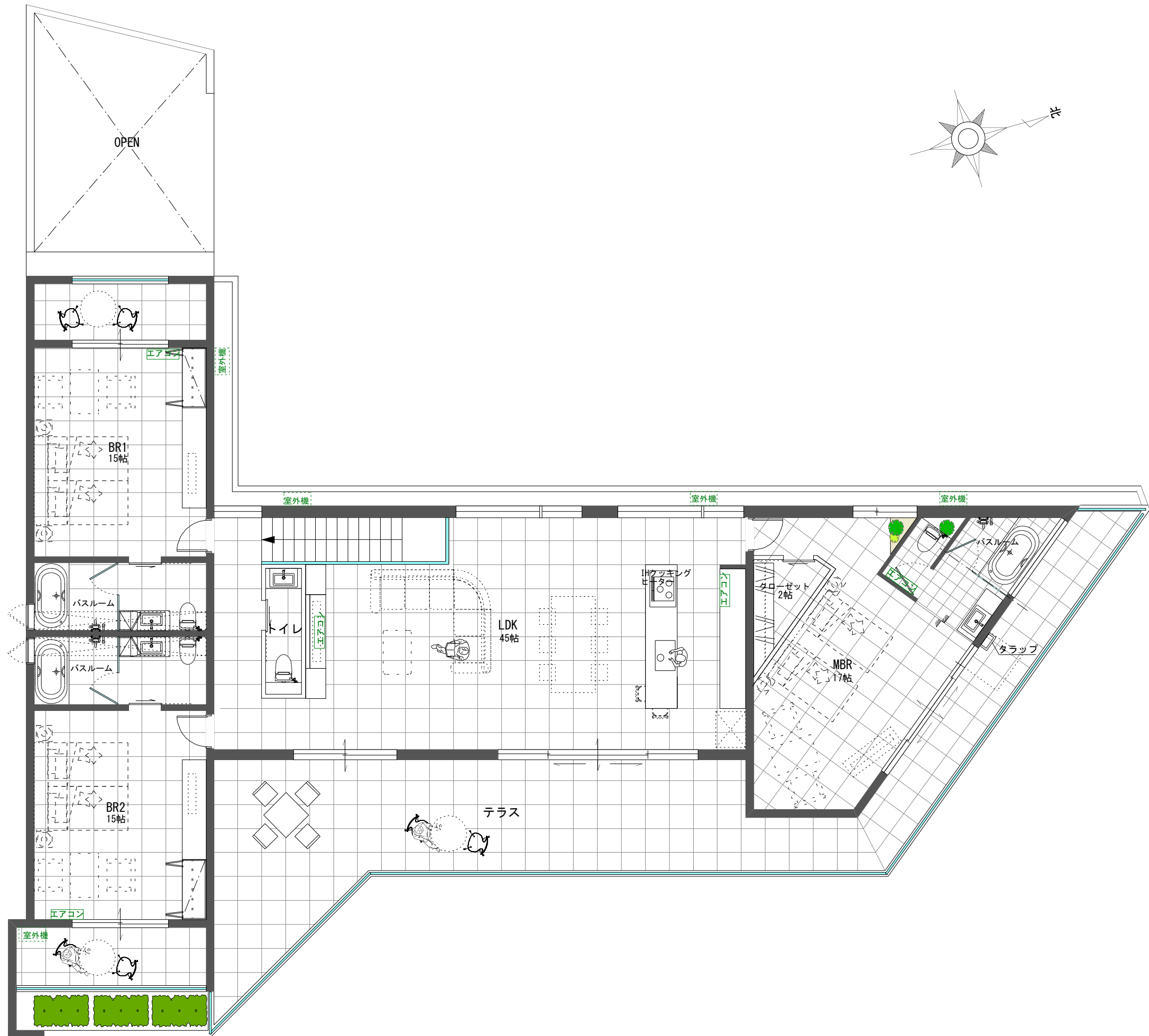
2階平面図
