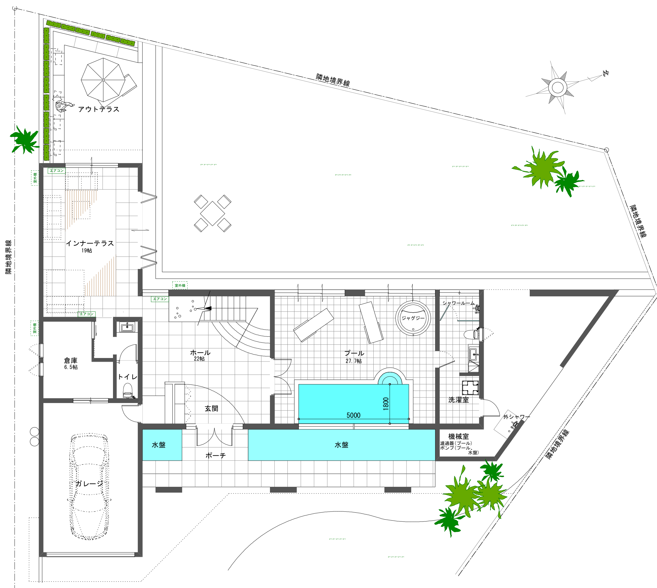
1階平面図
